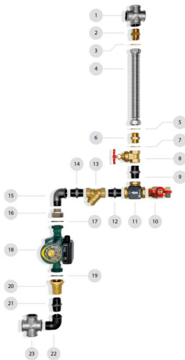
Rys nr 42. Zestaw hydrauliczny kotłów typu Smart Fire SF11 i SF15 1 ÷ 14 – jak na rys nr 41; 15-kolanko; 16-półśrubunek; 17-uszczelka gumowa; 18-pompa; 19-uszczelka gumowa; 20-półśrubunek z zaworem; 21-nypel; 22-kolanko; 23-czwórnik (przyłącze powrotu kotła);
