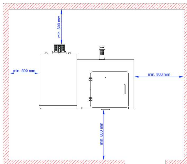
Rys nr 32. Przykład umiejscowienia kotła typu Smart Fire SF41 z zasobnikiem 440L w kotłowni
