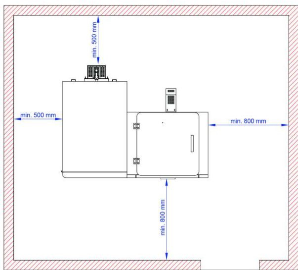
Rys nr 31. Przykład umiejscowienia kotła typu Smart Fire SF41 z zasobnikiem 240L w kotłowni
