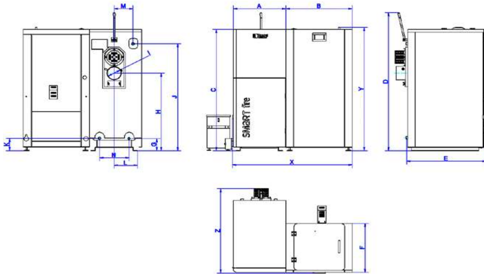
Rys nr 27. Wymiary kotłów Smart Fire SF31 oraz SF41 z zasobnikiem paliwa 240L i systemem automatycznego odpopielania
