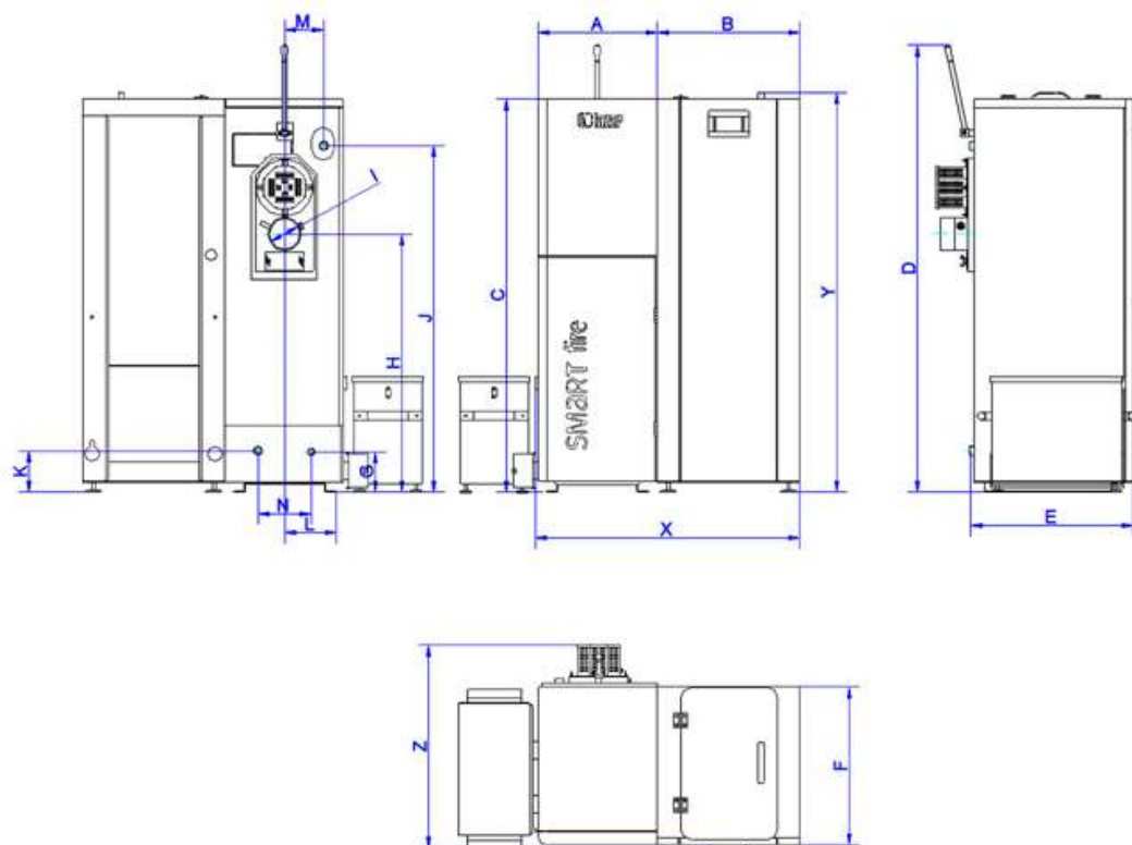
Rys nr 21. Wymiary kotłów Smart Fire SF11, SF15, SF15/3bar, SF22 oraz SF22/3bar z zasobnikiem paliwa 150L i systemem automatycznego odpopielania
