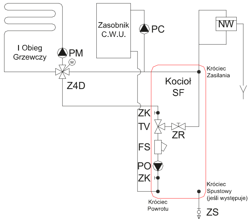
Rys nr 37. Układ otwarty + CWU < 220L 1 obieg na zaworze 4D
