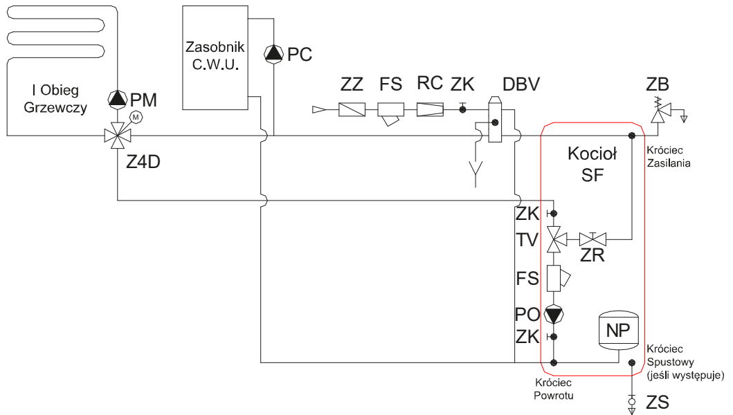
Rys nr 38. Układ zamknięty + CWU < 220 L + obieg na zaworze 4D
