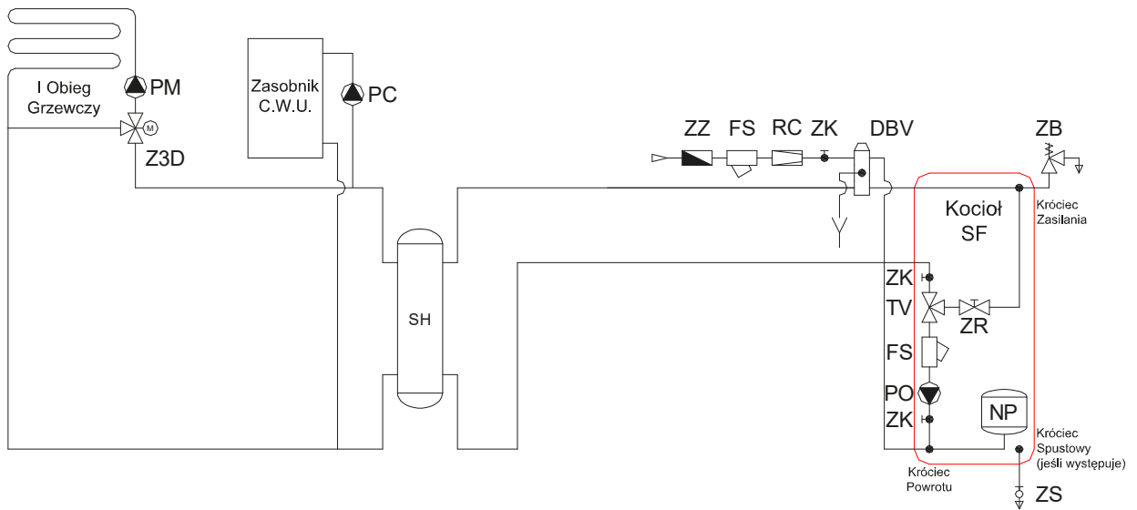
Rys nr 35. Układ zamknięty + CWU > 220L + 1 obieg na zaworze 3D
