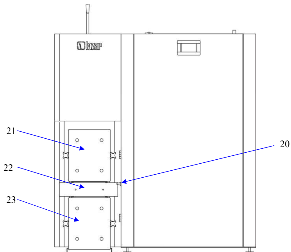
Rys nr 6. Opis schematyczny kotłów typu Smart Fire SF 11, SF15, SF15/3bar, SF22, SF22/3bar, SF31 oraz SF41 20-wyłącznik krańcowy maskownicy drzwi kotła; 21-drzwi komory palnika; 22-maskownica zapalarki ceramicznej oraz wyczystki palnika; 23-drzwi komory popielnika;
