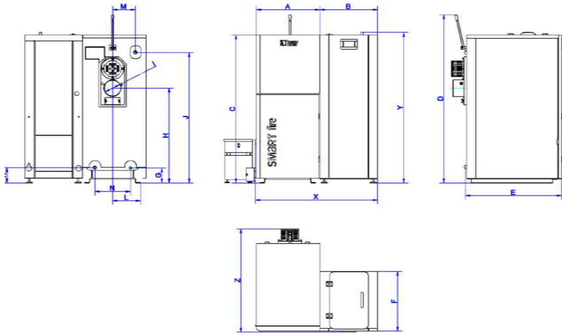
Rys nr 26. Wymiary kotłów Smart Fire SF31 oraz SF41 z zasobnikiem paliwa 150L i systemem automatycznego odpopielania
