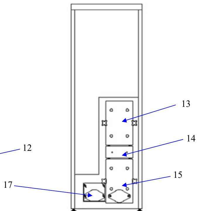
12-pokrywa otworu rewizyjnego; 13-drzwi komory spalania; 14-maskownica zapalarki ceramicznej oraz wyczystki palnika; 15-drzwi komory popielnika; 16-pokrywa otworu rewizyjnego czopucha spalinowego; 17-wyczystka dolnej części wymiennika ciepła;
