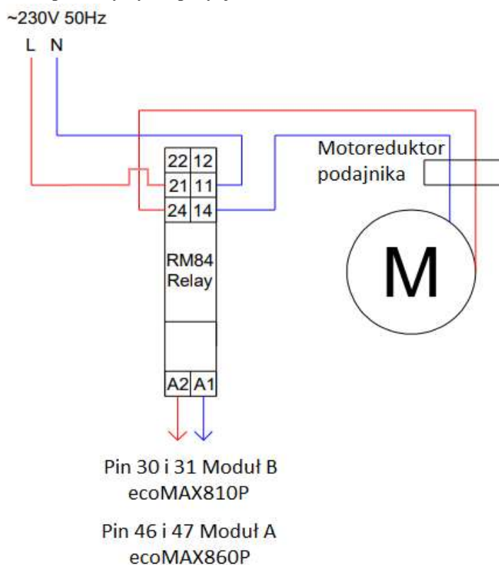
Rys nr 20. Schemat podłączenia systemu automatycznego odpopielania do regulatora kotła.
