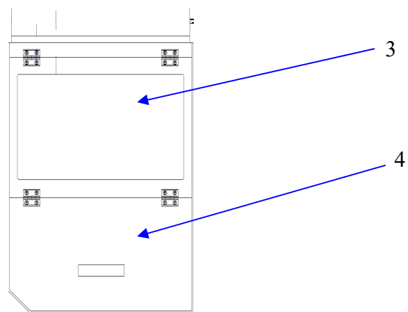
Rys nr 11. Opis schematyczny kotła Smart Fire SF11/45L 1-panel wyświetlacza dotykowego; 2-maskownica; 3-pokrywa rewizyjna; 4 - klapa zasobnika paliwa;
