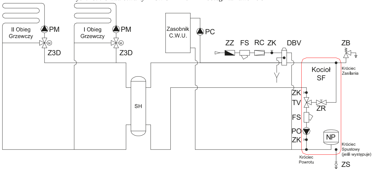
Rys nr 40. Układ zamknięty + CWU < 220L + 2 obiegi na zaworze 3D
