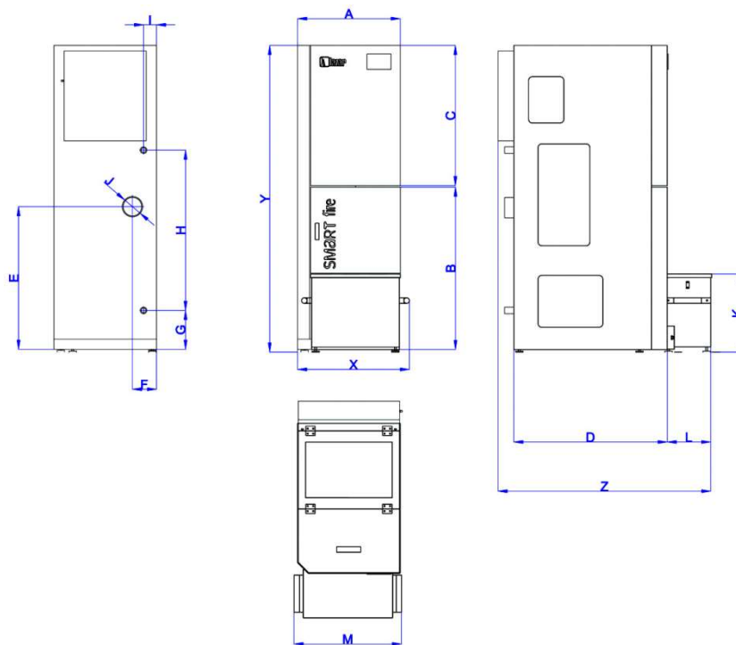
Rys nr 24. Wymiary kotła Smart Fire SF11 z zasobnikiem paliwa 130L i systemem automatycznego odpopielania
