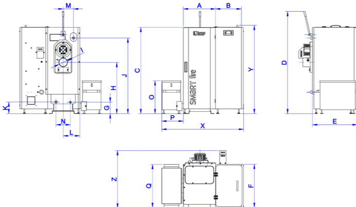
Rys nr 29. Wymiary kotłów Smart Fire SF11 COMPACT oraz SF15 COMPACT z systemem automatycznego odpopielania
