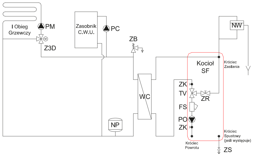
Rys nr 36. Układ z płytowym wymiennikiem ciepła – kocioł w układzie otwartym, wymiennik CWU i obieg grzewczy w układzie zamkniętym
