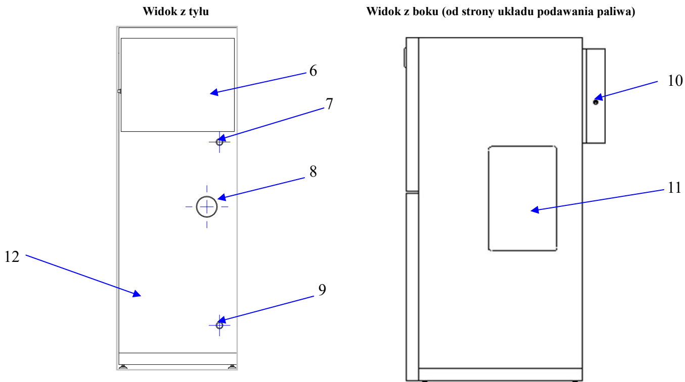
Rys nr 9. Opis schematyczny kotła Smart Fire SF11/130L 6-skrzynka elektryczna; 7-króciec zasilania; 8-czopuch spalinowy wraz z czujnikiem temperatury spalin oraz sondą Lambda (wyposażenie opcjonalne); 9-króciec wody powrotnej; 10-reset termostatu bezpieczeństwa STB (pod plastikową nakrętką); 11-pokrywa otworu rewizyjnego śluzy; 12-tylna maskownica;
