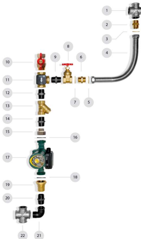
Rys nr 43. Zestaw hydrauliczny kotłów typu Smart Fire SF15/3bar, SF22, SF22/3bar, SF31 oraz SF41: 1-czwórnik (przyłącze zasilania kotła); 2-nypel mosiężny; 3-uszczelka twarda; 4-Przewód elastyczny EMICASA; 5-uszczelka twarda; 6-nypel mosiężny; 7-uszczelka twarda; 8-zawór zasuwowy (kryzujący); 9-nypel; 10-zawór kulowy (przyłącze powrotu instalacji); 11-zawór termostatyczny TV 55°C; 12-nypel; 13-filtr; 14-nypel; 15-półśrubunek; 16-uszczelka gumowa; 17-pompa; 18-uszczelka gumowa; 19-półśrubunek z zaworem; 20-nypel; 21-kolanko; 22-czwórnik (przyłącze powrotu kotła);
