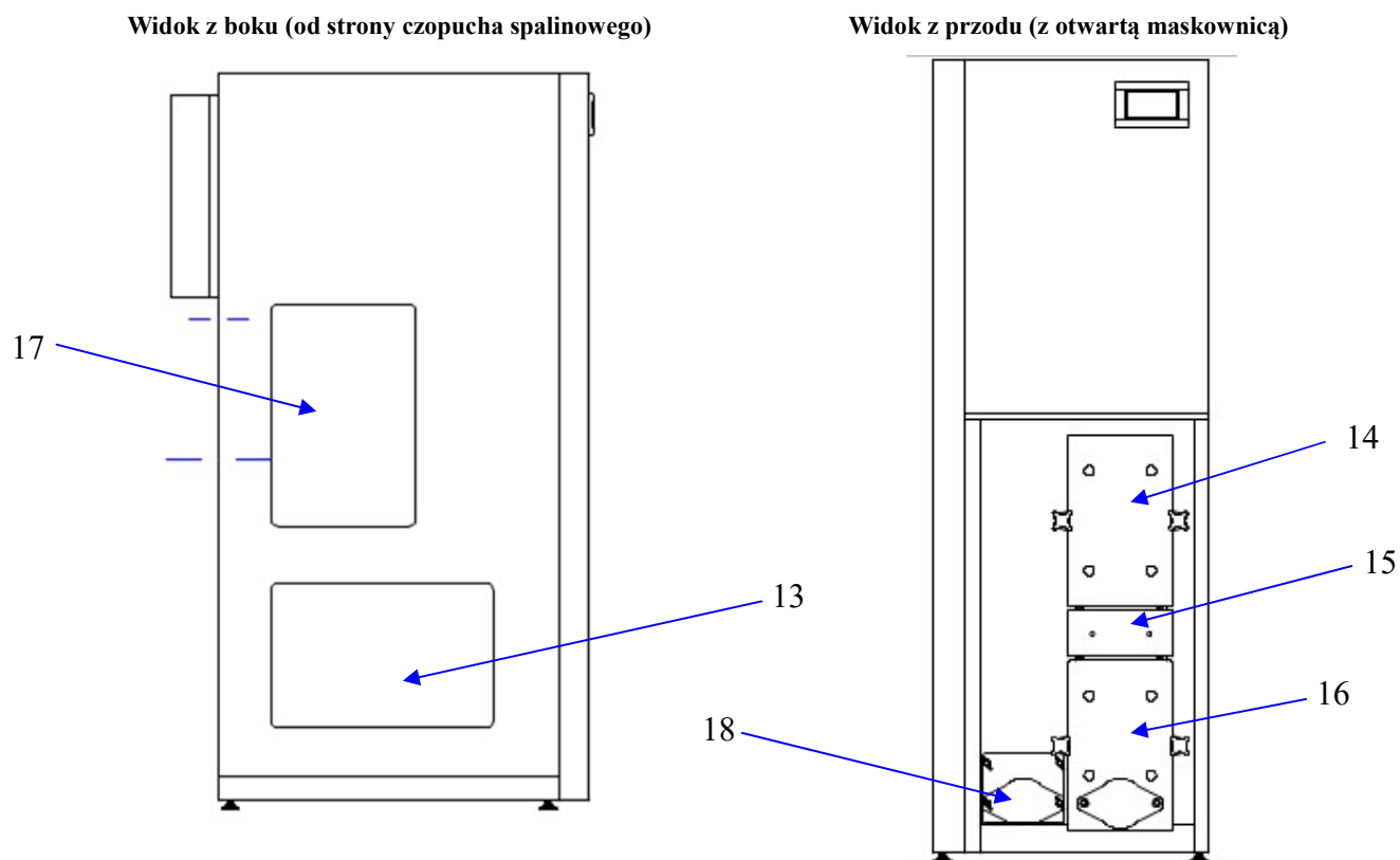
13-pokrywa otworu rewizyjnego; 14-drzwi komory spalania; 15-maskownica zapalarki ceramicznej oraz wyczystki palnika; 16-drzwi komory popielnika; 17-pokrywa otworu rewizyjnego czopucha spalinowego; 18-wyczystka dolnej części wymiennika ciepła;
