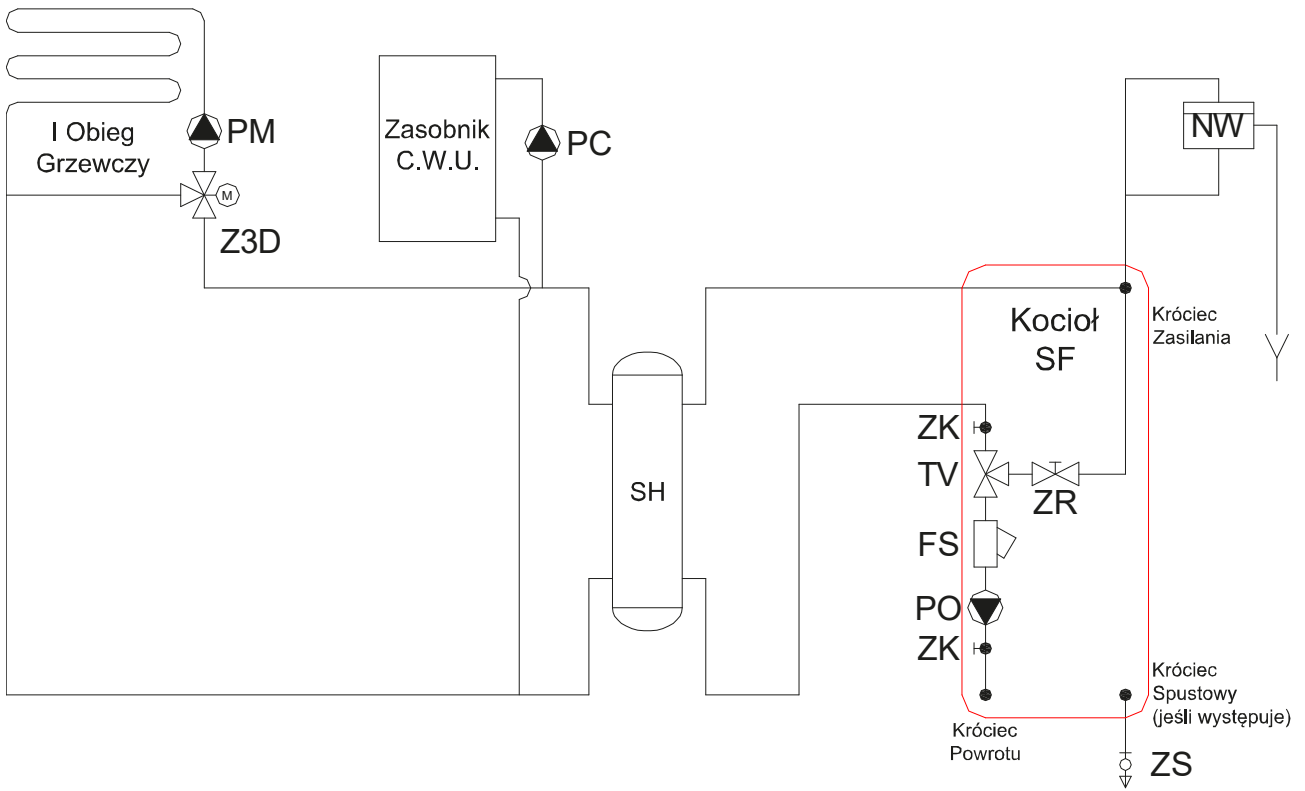
Rys nr 34. Układ otwarty + CWU > 220L + 1 obieg na zaworze 3D
