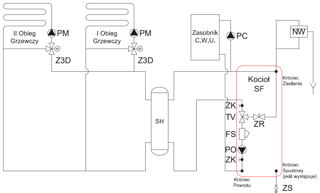
Rys nr 39. Układ otwarty + CWU < 220L + 2 obiegi na zaworze 3D
