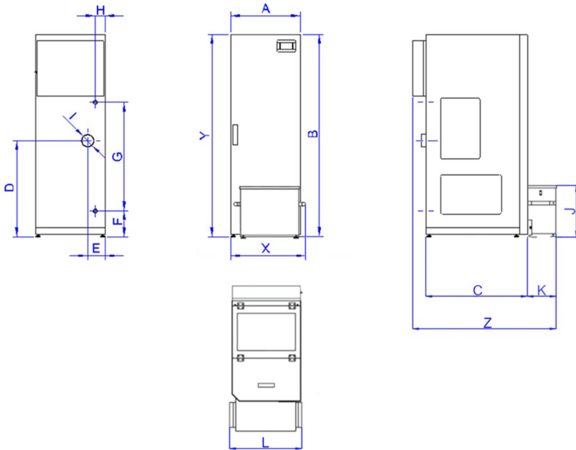
Rys nr 25. Wymiary kotła Smart Fire SF11 z zasobnikiem paliwa 45L i systemem automatycznego odpowielania
