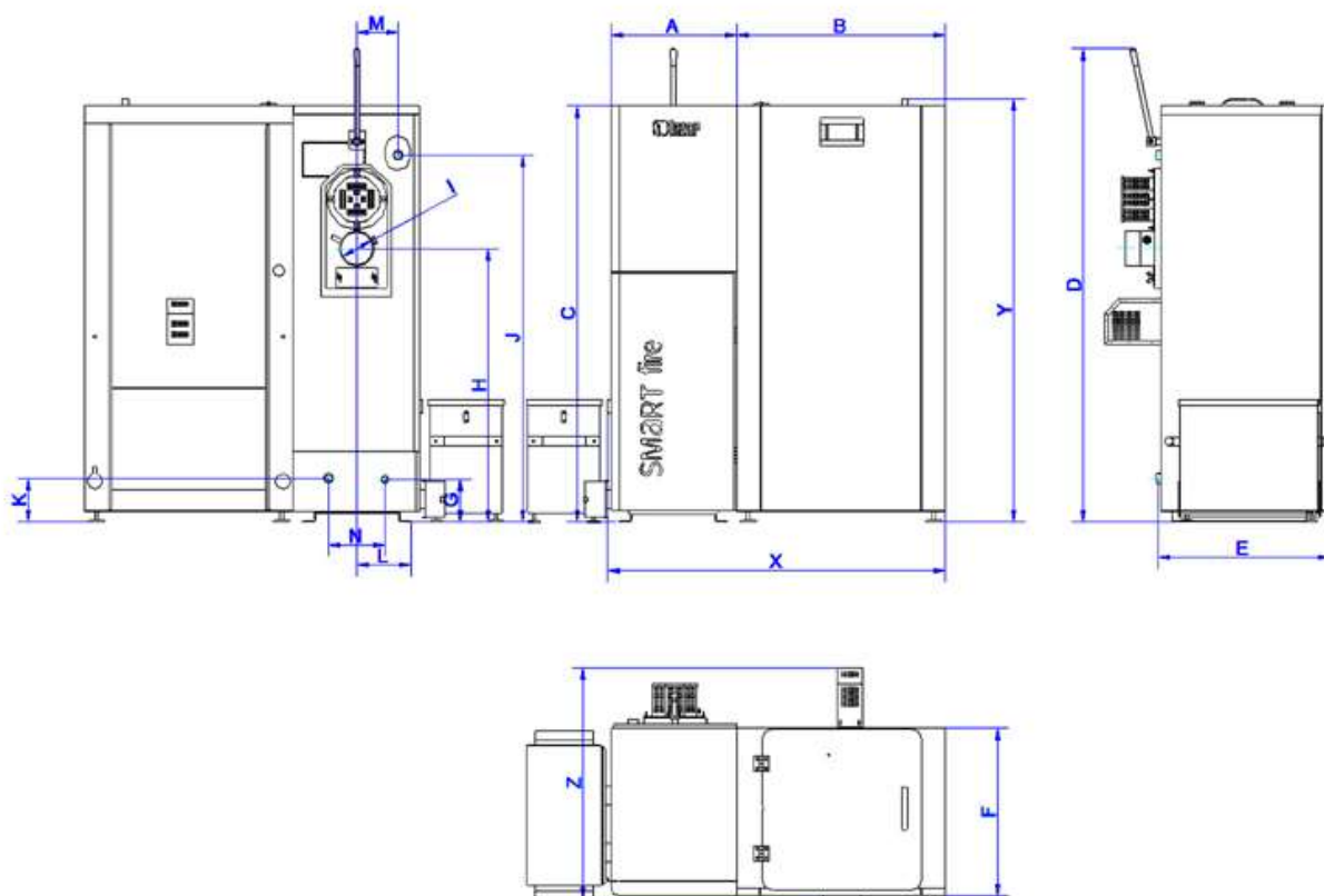
Rys nr 22. Wymiary kotłów Smart Fire SF11, SF15, SF15/3bar, SF22 oraz SF22/3bar z zasobnikiem paliwa 240L i systemem automatycznego odpopielania
