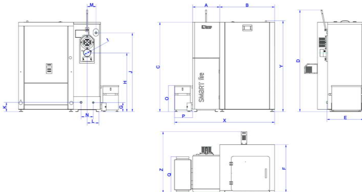
Rys nr 23. Wymiary kotłów Smart Fire SF11, SF15, SF15/3bar, SF22 oraz SF22/3bar z zasobnikiem paliwa 440L i systemem automatycznego odpowielania
