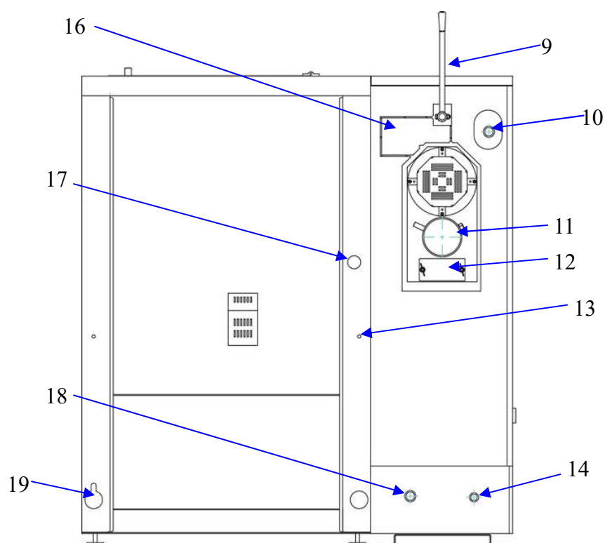
Rys nr 5. Opis schematyczny kotłów typu Smart Fire SF 11, SF15, SF15/3bar, SF22, SF22/3bar, SF31 oraz SF41:
